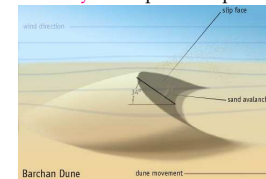
FIG. 1 – Schéma d'une Barkhane, Wikipédia 2007
