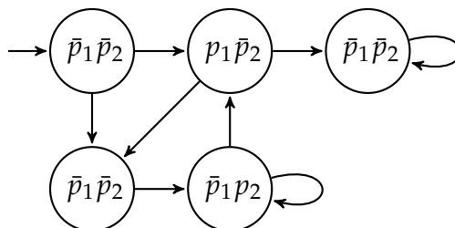
FIG. 1 – Structure de Kripke. Elle sert telle quelle dans l'exercice 1 ; puis vous devrez la modifier dans l'exercice 2
