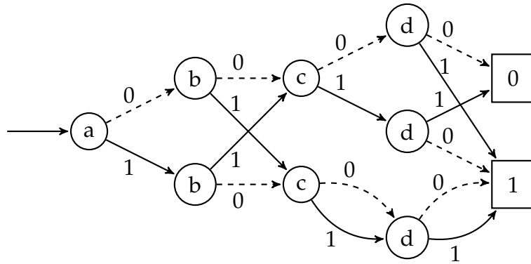
FIG. 2 – Diagramme de décision binaire, utilisé dans l'exercice 5.
